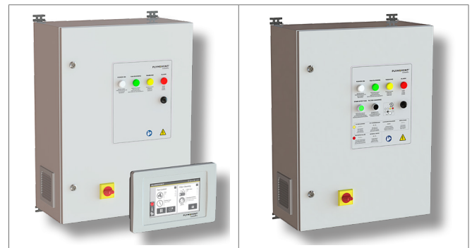
SCS-Diluter PRO mit ControlPro: intelligente Steuer- + Regelungseinheit mit HMI für umfangreiche Ventilator-/ Filteransteuerungsfunktionen; Fernzugriff über Netzwerk
